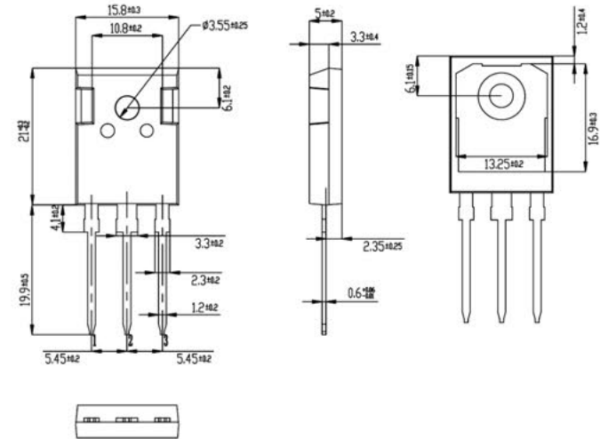
TO-247-3L
